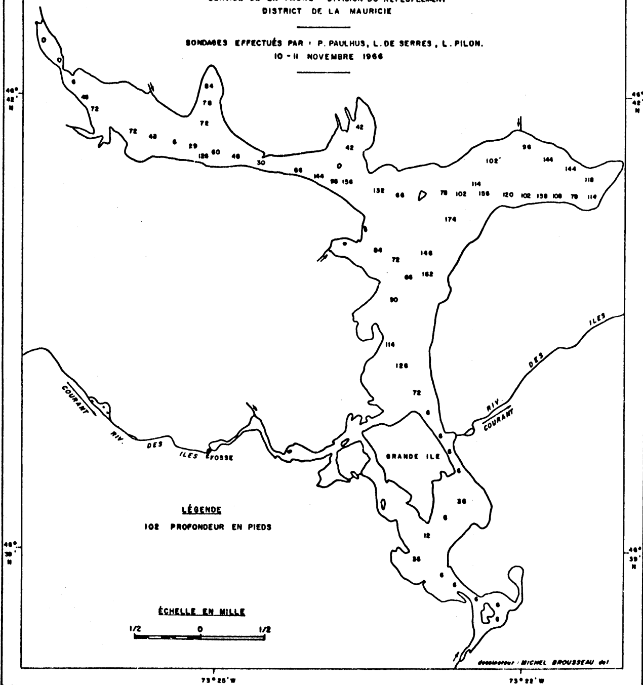
FIGURE 3. CARTE BATHYMETRIQUE DU LAC SORCIER.
